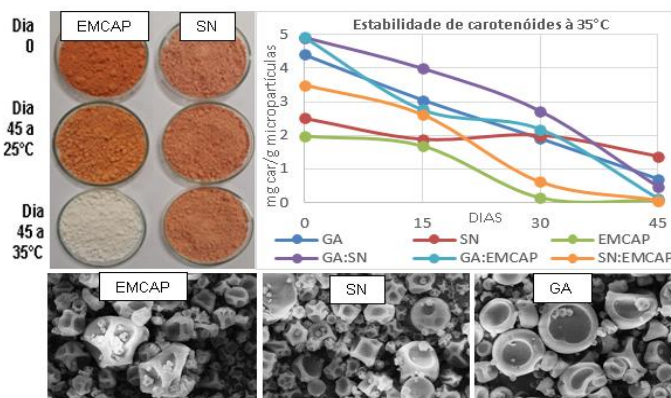
Figura 1. Estabilidade de cor e carotenoides ao longo do tempo, e microscopia eletrônica de varredura.
